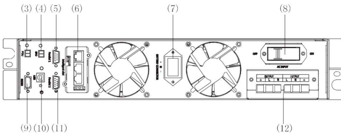
Задняя панель
